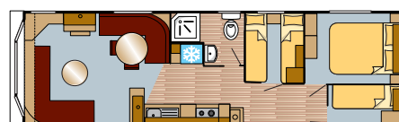
32'x10' 3 Bed
